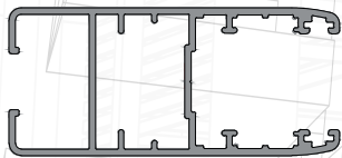
G-3705 - 1.364 kg/m 101576 - 1.840 kg/m
