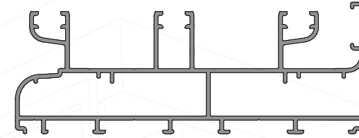
G-3702 - 2.574 kg/m 101576 - 1.840 kg/m
